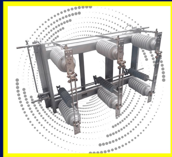
SECCIONADOR TRIPOLAR 17.5 / 36 / 52 kV 630 / 1250 A
