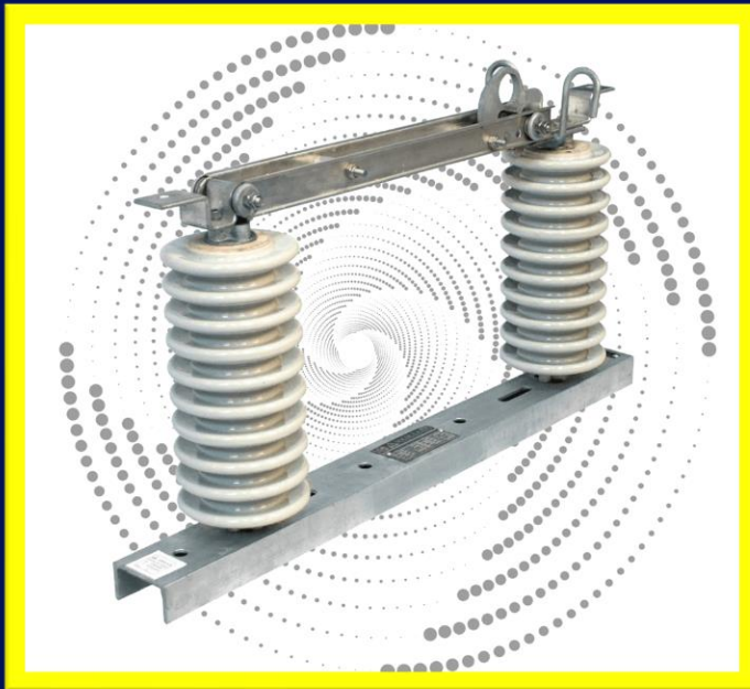
SECCIONADOR MONOPOLAR 15 / 36 / 46 kV 400 / 600 A
